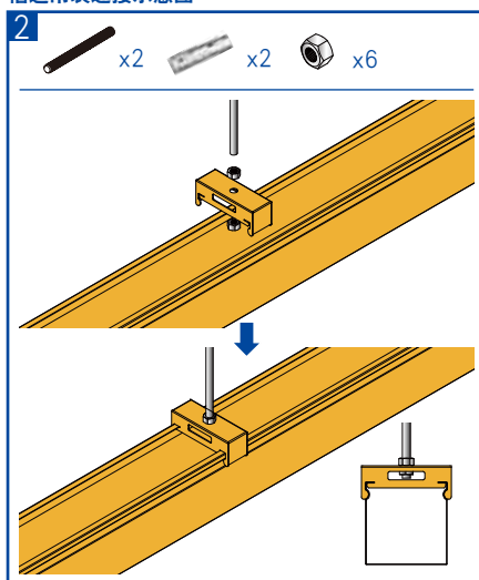
变径接板连接示意图
