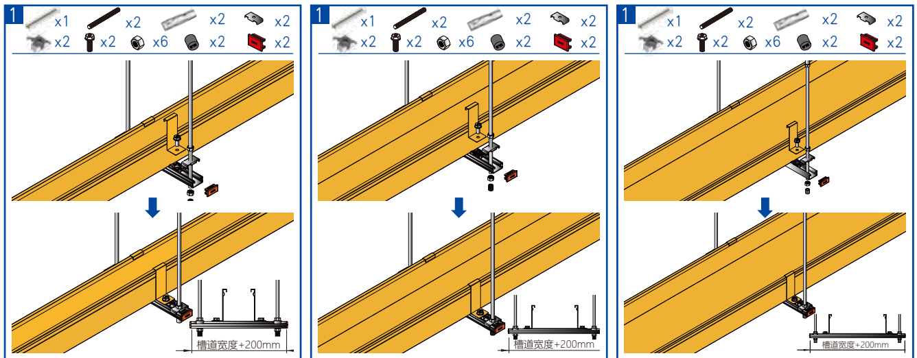
槽道吊装连接示意图
