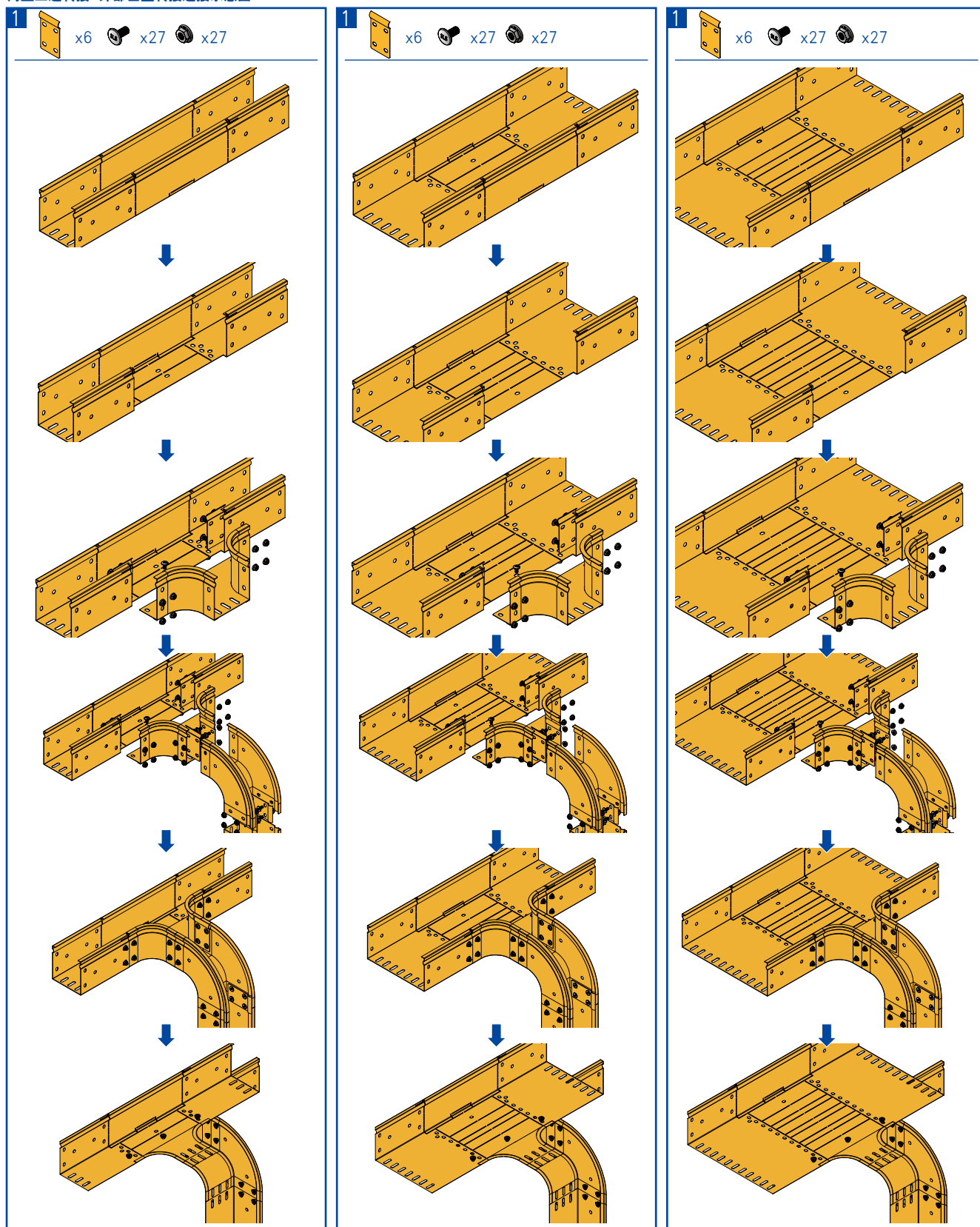
内置三通转接+外部垂直转接连接示意图
