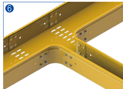
6 三通变径转接：用来提供不同宽度直线段的3方向分支
