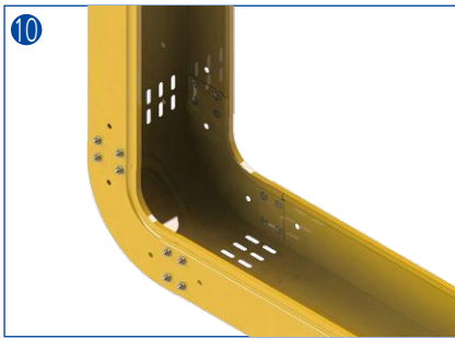
内部垂直转接：用来提供垂直方向内部90度转接
