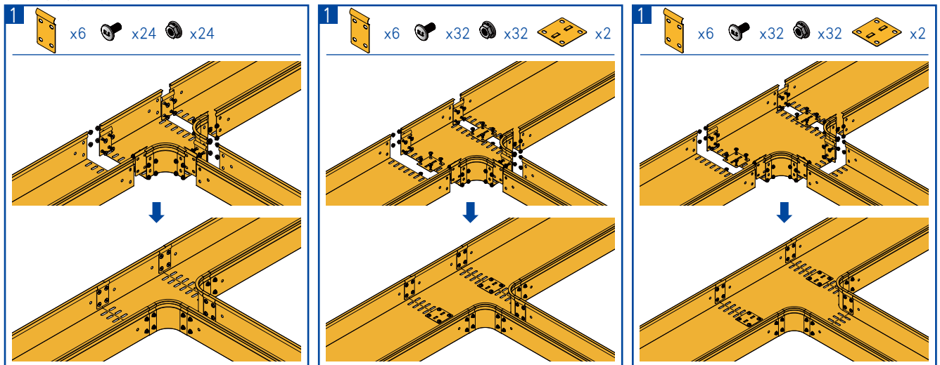
四通转接连接示意图
