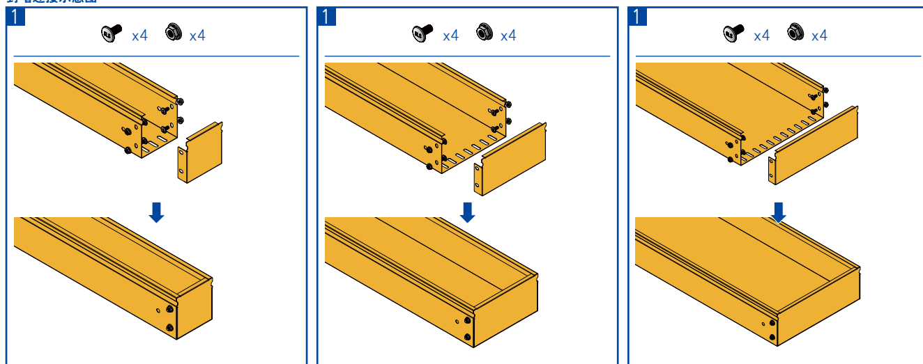
封堵连接示意图
