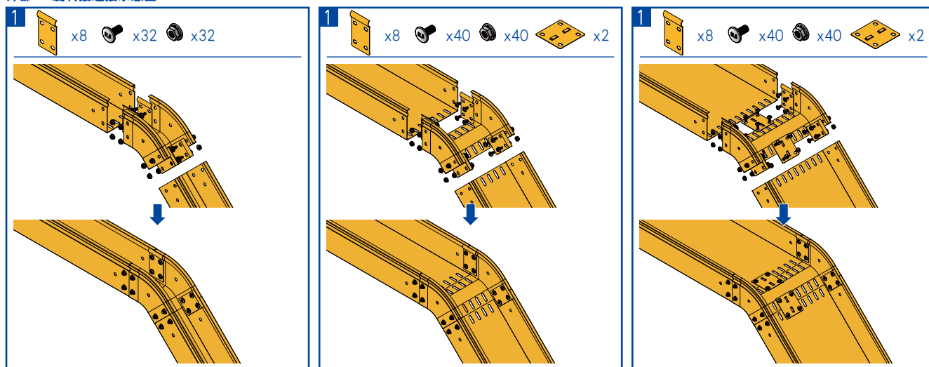
内部135度转接连接示意图
