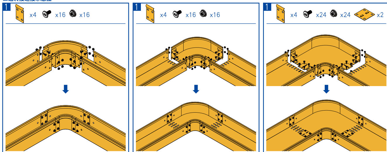
二通转连接示意图
