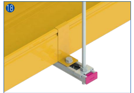
侧面固定夹：用于SFS光纤槽道横担固定
