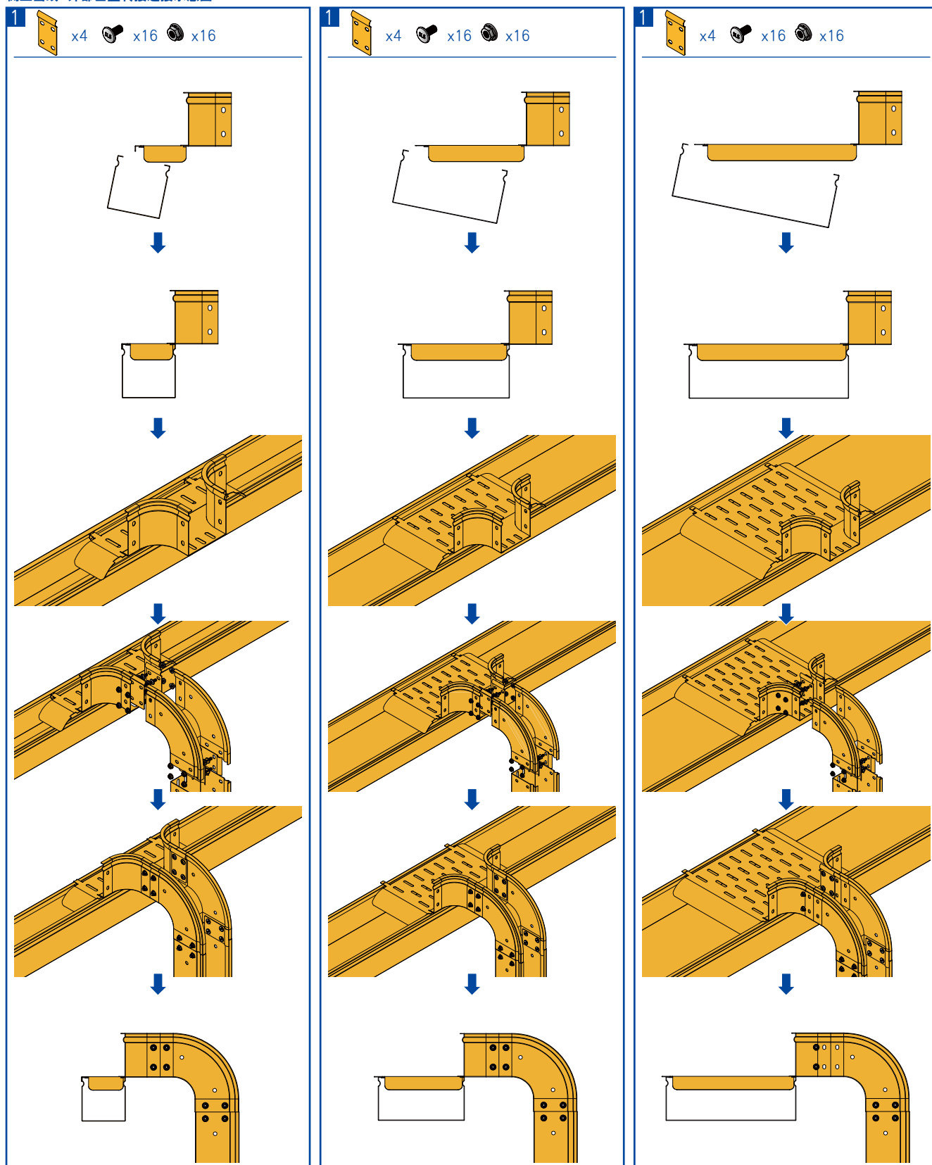
侧上出线+外部垂直转接示意图
