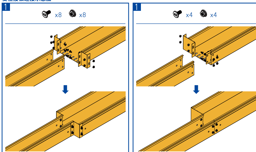
变径接板连接示意图
