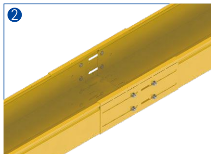
2 伸缩段：用于直通段补偿，可调节不同长度
