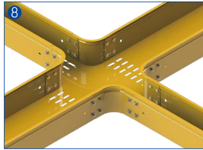
四通变径转接：用来提供不同宽度直线段的四方向分支
