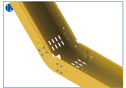
内部135度转接：用来提供垂直方向内部135度转接
