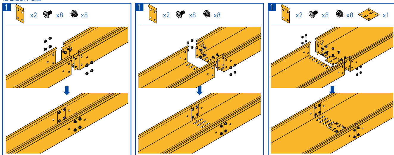
伸缩段连接示意图
