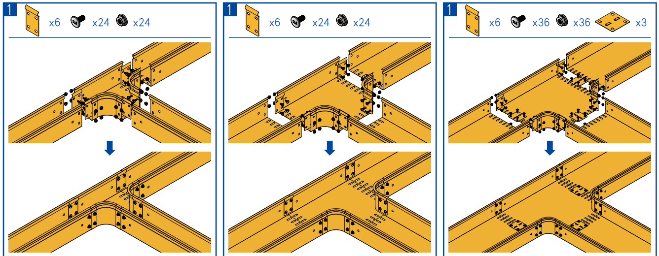
三通变径转接连接示意图
